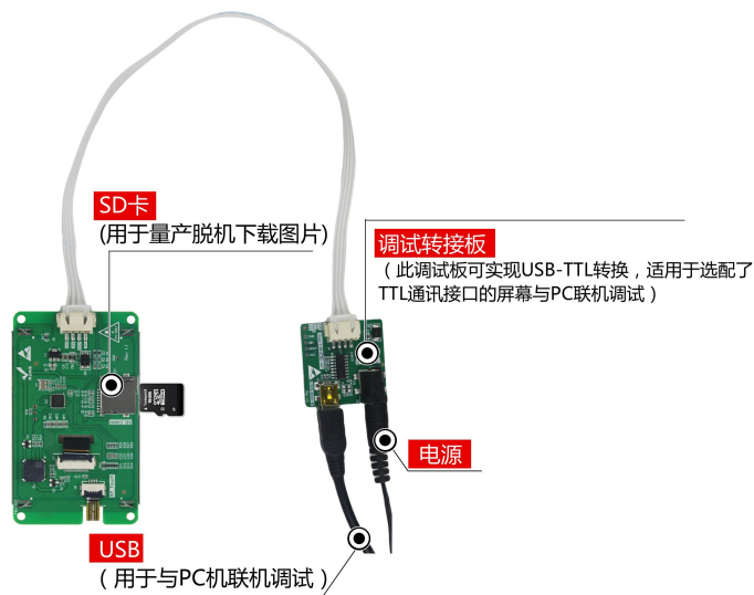
图 1-4 调试工具图
